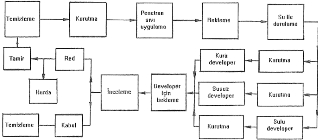
Şekil 4. Su ile yıkanabilir penetranla yapılan muayenenin akış diyagramı [2]
